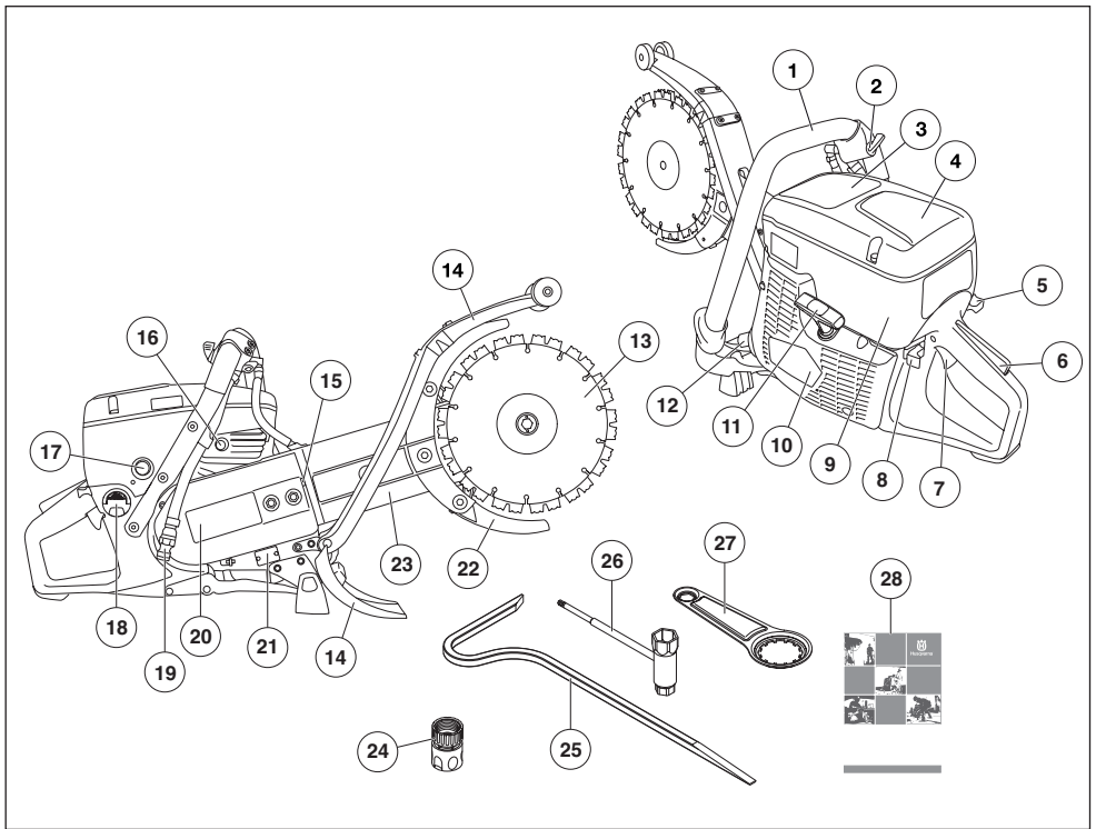
切割锯 K760 Cut-n-Break 上的零组件图示说明
